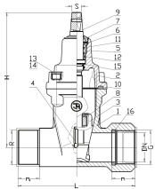
Mittakuva_sk_uk_venttiili_Durapu sh_DN50
